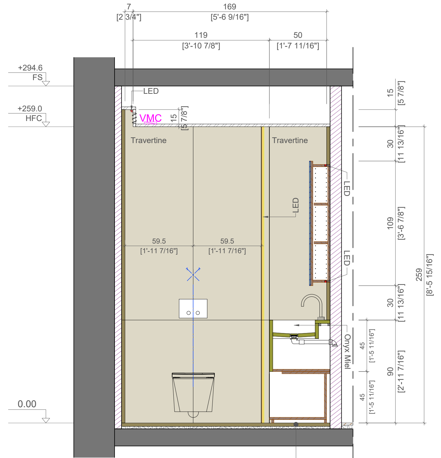
ELEVATION BB
